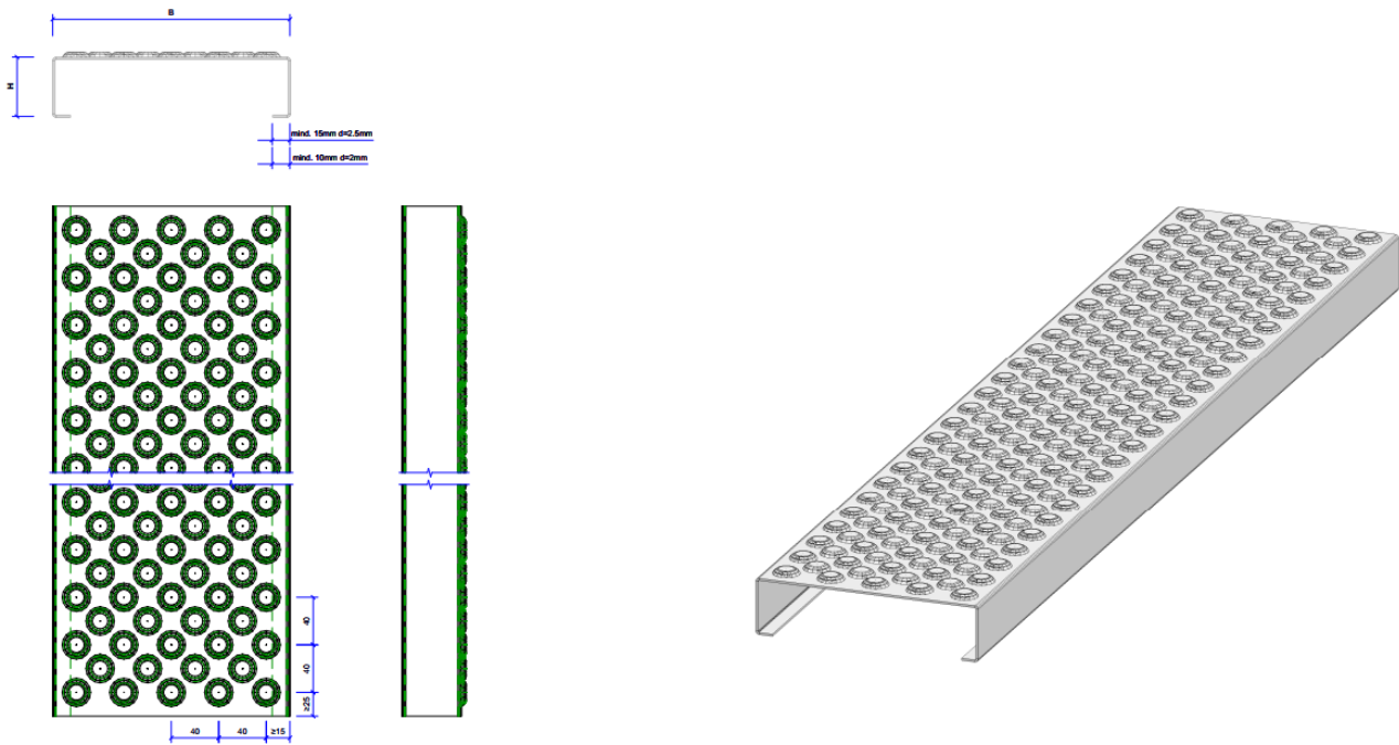
Symbolbild Vermassung
